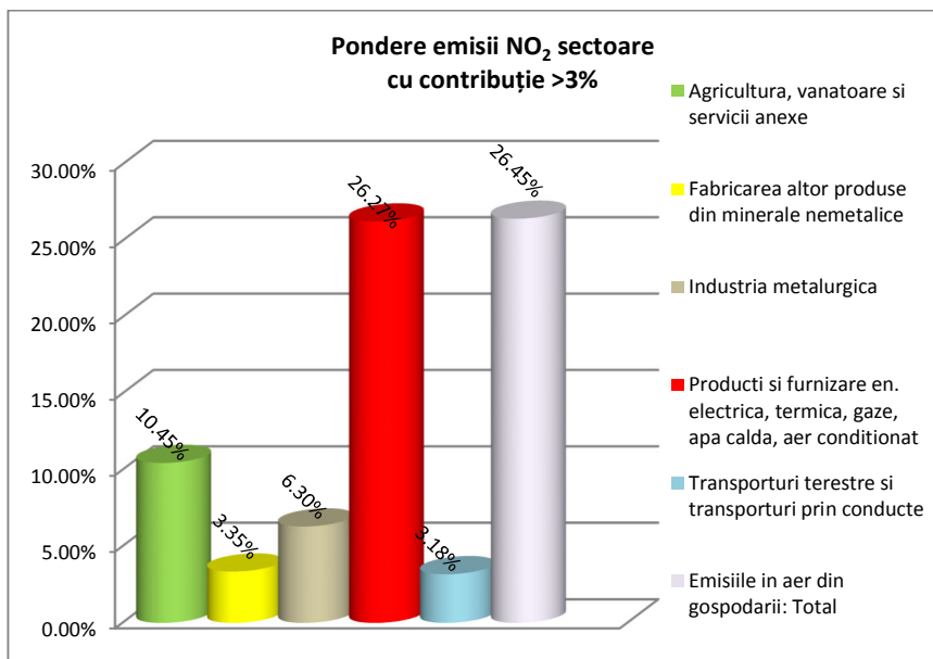
Figura nr. 50. Pondere emisii NO 2 pe sectoare de activitate
