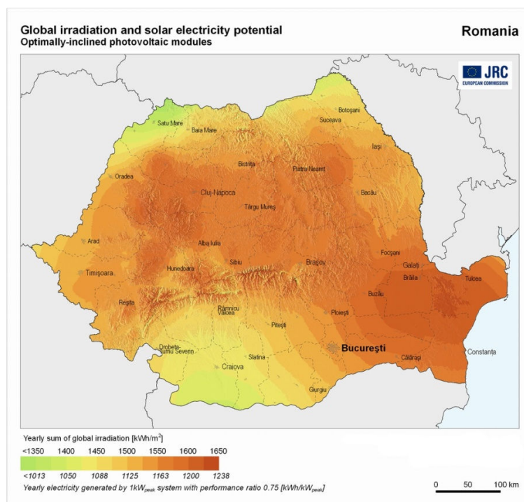
Figura nr.10. Harta radiației solare anuale
