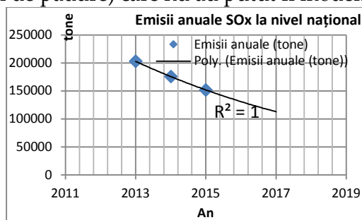
Figura nr. 24. Tendința de evoluție a emisiilor SO 2 la nivel național
