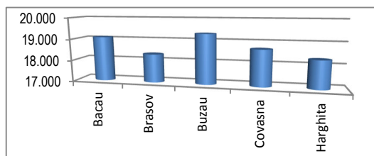
Figura nr. 35. Concentrații fond regional PM 10 anul 2016
