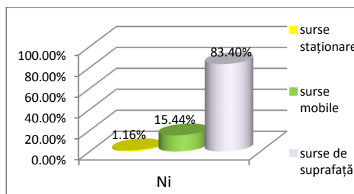
Figura nr. 47. Alocare emisii totale Ni pe tipuri de surse
