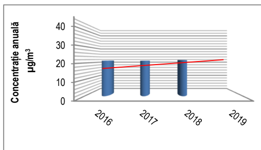
Figura nr. 15. Evoluție concentrații anuale PM10 2016-2018
