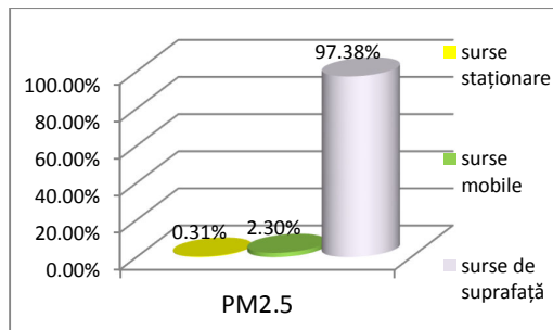
Figura nr. 39. Alocare emisii totale PM 2.5 pe tipuri de surse
