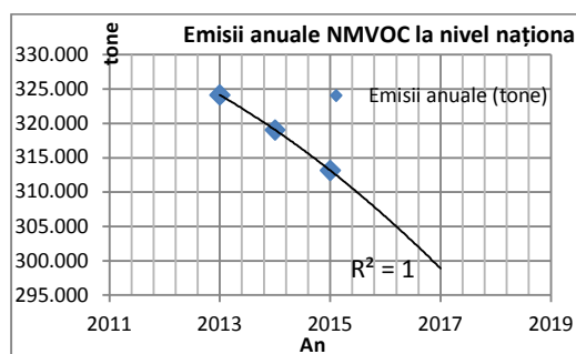
Figura nr. 26. Tendință emisii la nivel național
