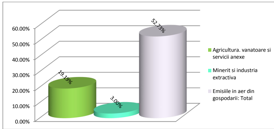
Figura nr. 53. Pondere emisii NMVOC pe sectoare de activitate
