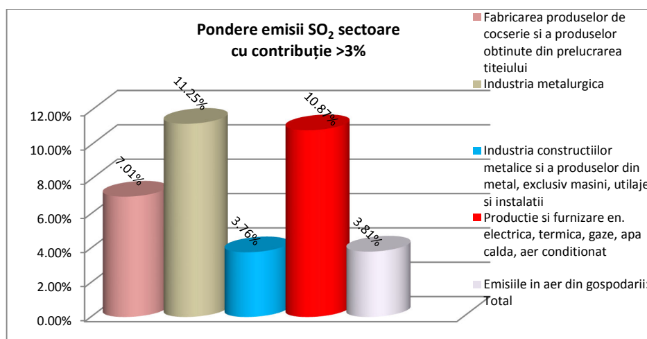
Figura nr. 51. Pondere emisii SO 2 pe sectoare de activitate
