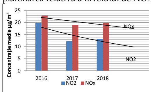
Figura nr. 19. Tendința concentrații medii anuale \text{NO}_2
