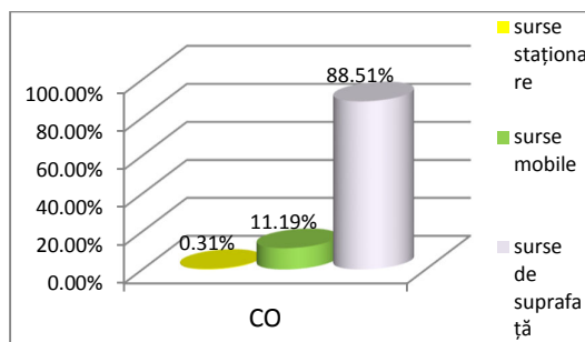
Figura nr.41. Alocare emisii totale CO pe tipuri de surse
