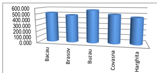
Figura nr. 32. Concentrații fond regional CO anul 2016
