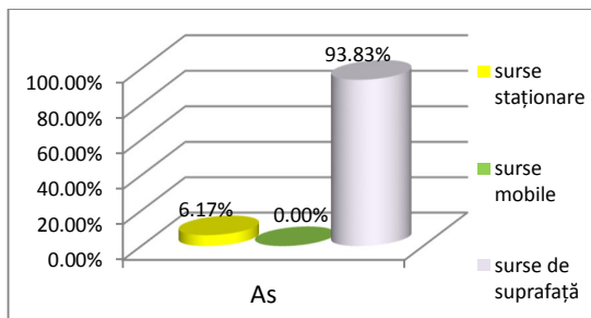
Figura nr. 44. Alocare emisii totale As pe tipuri de surse
