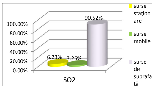
Figura nr.42. Alocare emisii totale SO2 pe tipuri de surse
