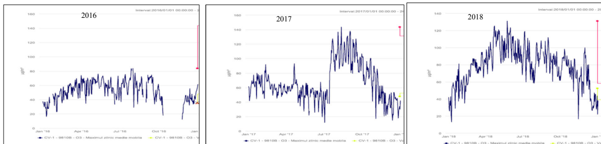
Figura nr. 63. Maximum zilnic al mediei mobile O 3 (Sursa: www.calitateaer.ro)
