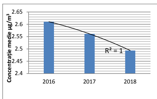
Figura nr. 25. Tendință concentrații medii anuale de benzen
