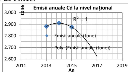
Figura nr. 28. Tendință emisii Cd la nivel național
