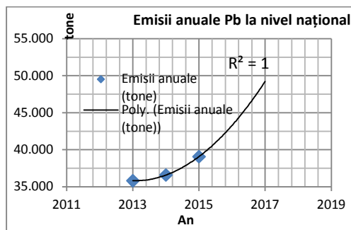
Figura nr. 30. Tendință emisii Pb la nivel național.
