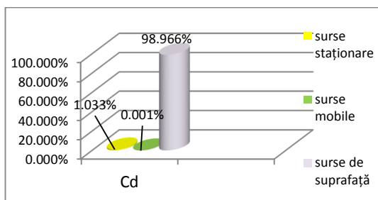
Figura nr. 46. Alocare emisii totale Cd pe tipuri de surse
