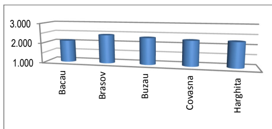
Figura nr. 31. Concentrații fond regional SO 2 anul 2016
