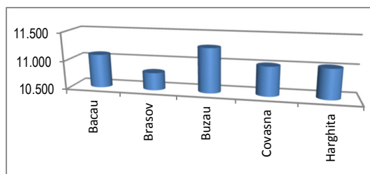
Figura nr. 34. Concentrații fond regional NO x anul 2016
