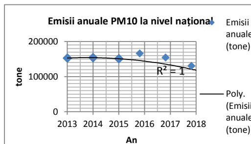
Figura nr. 16. Tendința de evoluție a emisiilor PM10 la nivel național
