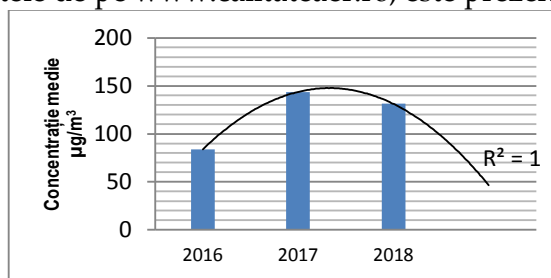
Figura nr. 64. Evoluția concentrațiilor O 3 - maxim zilnic al mediilor pe 8 ore anii 2016 - 2018
