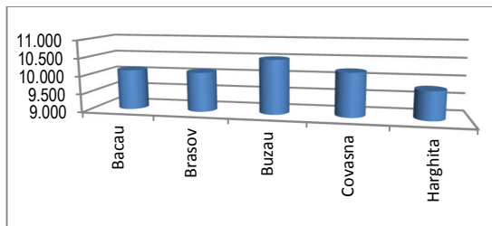
Figura nr. 33. Concentrații fond regional NO 2 anul 2016
