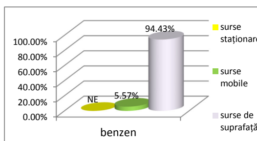
Figura nr.43. Alocare emisii totale benzen pe tipuri de surse
