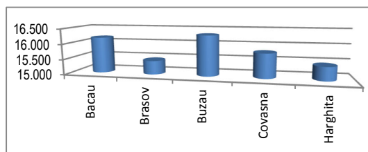
Figura nr. 36. Concentrații fond regional PM 2.5 anul 2016
