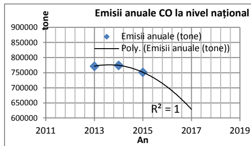
Figura nr. 22. Tendința de evoluție a emisiilor CO
