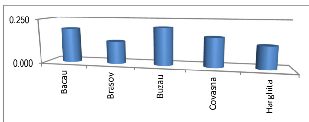
Figura nr. 37. Concentrații fond regional benzen anul 2016
