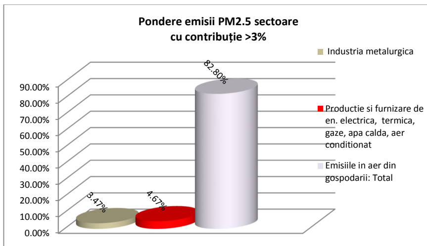
Figura nr. 49. Pondere emisii PM2.5 pe sectoare de activitate
