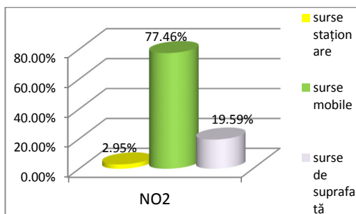
Figura nr. 40. Alocare emisii totale NO2 pe tipuri de surse
