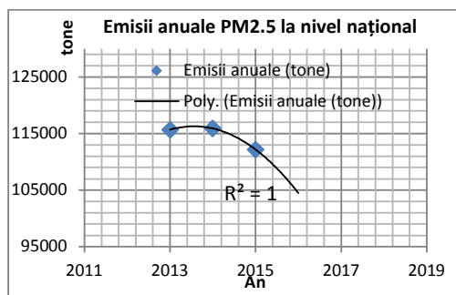
Figura nr. 18. Tendința de evoluție a emisiilor PM2,5 la nivel național
