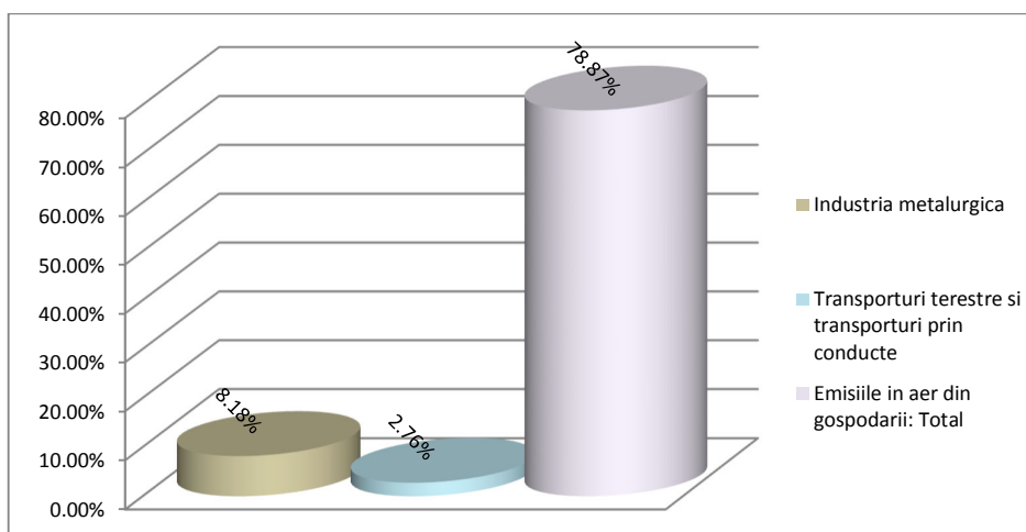
Figura nr. 52. Pondere emisii CO pe sectoare de activitate
