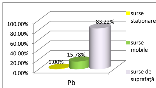
Figura nr. 45. Alocare emisii totale Pb pe tipuri de surse
