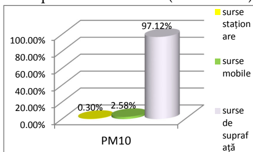
Figura nr.38. Alocare emisii totale PM10 pe tipuri de surse
