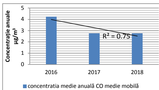
Figura nr. 21. Tendința concentrații anuale CO
