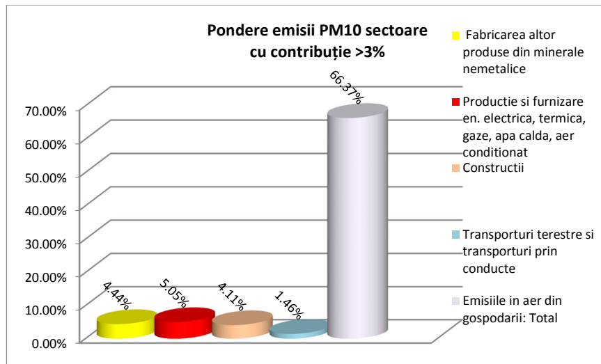
Figura nr. 48. Pondere emisii PM10 pe sectoare de activitate
