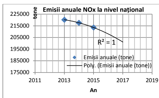
Figura nr. 20. Tendința de evoluție a emisiilor \text{NO}_x la nivel național
